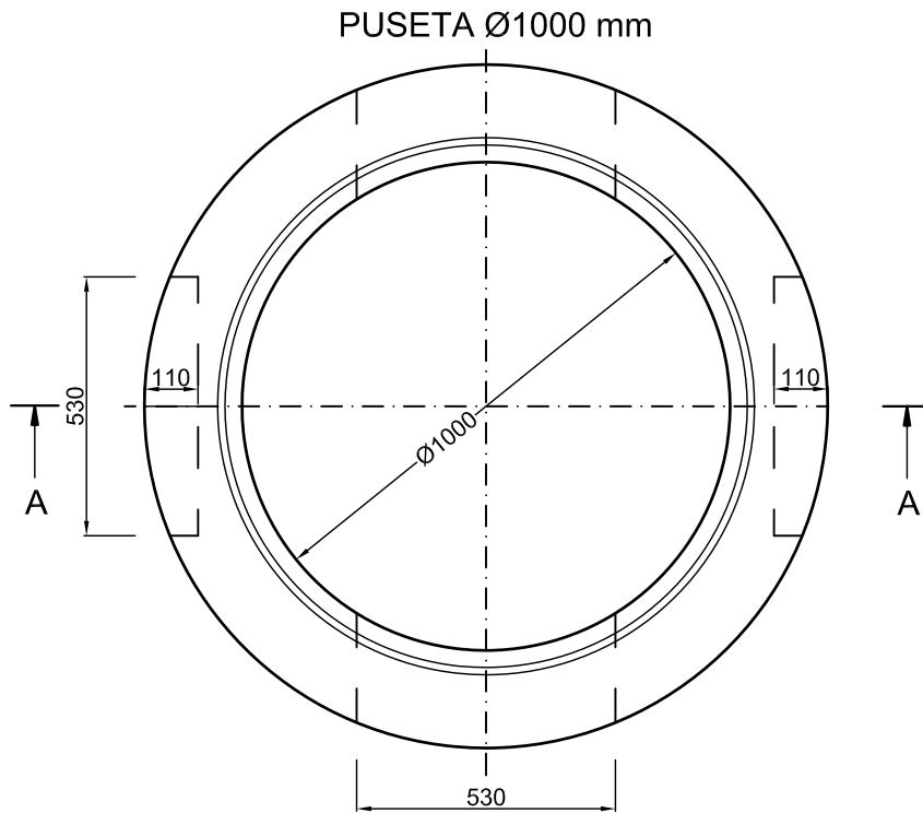
PRERJA A-A
